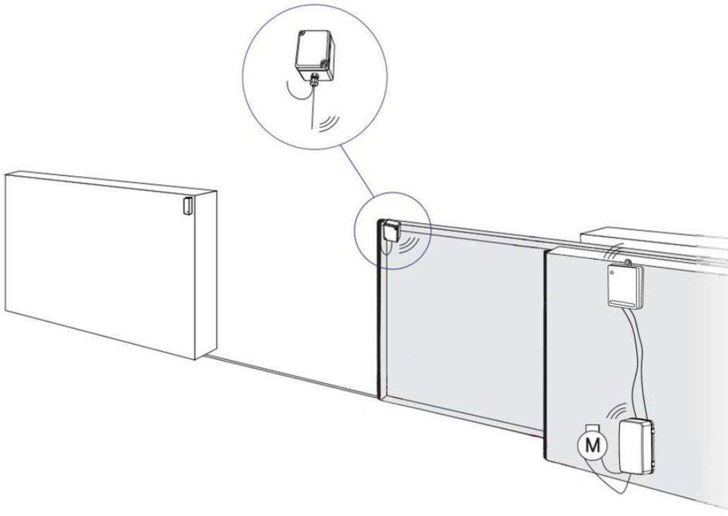
Şekil 9 - Yana Kayar Bahçe Kapılarında Kullanım
