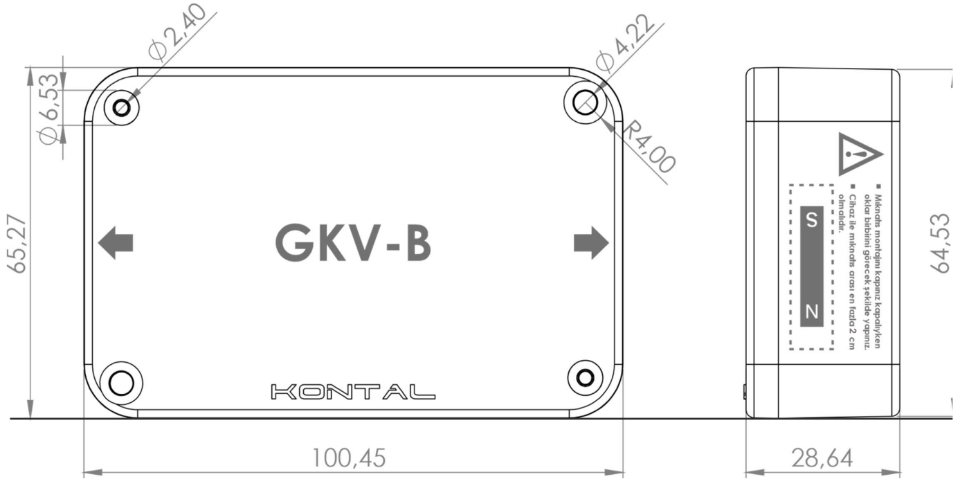
Şekil 17 - GKV-B Boyutlar
