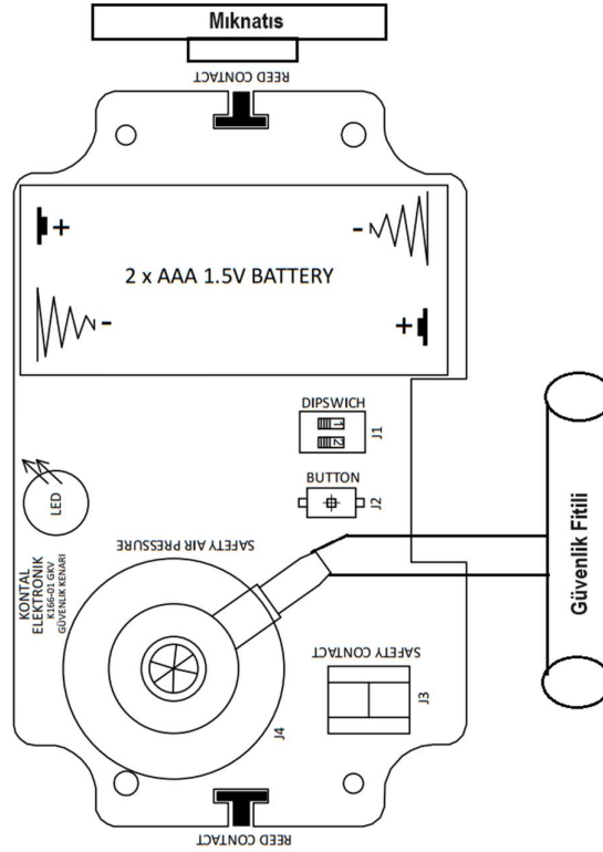
Şekil 11 – GKV-B Bağlantı Şeması
