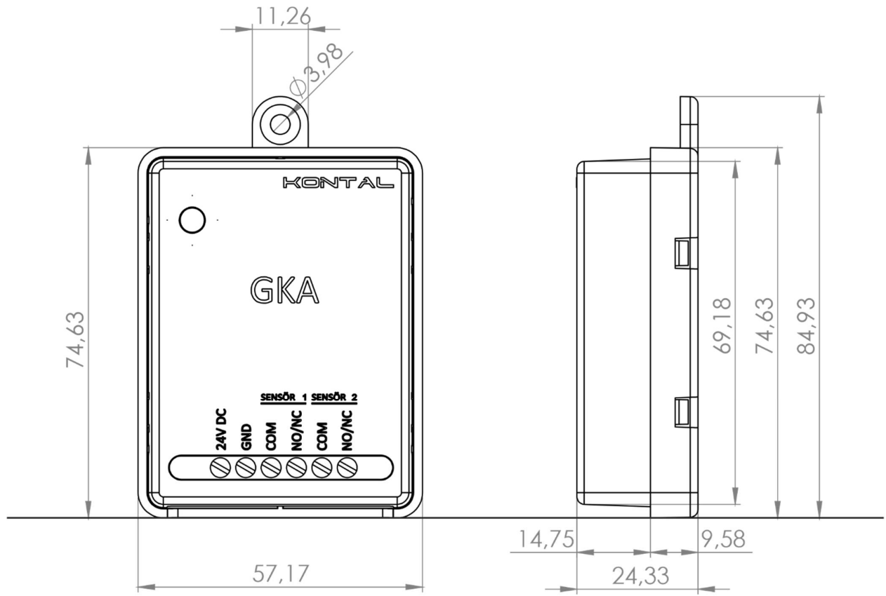
Şekil 16 - GKA Boyutlar
