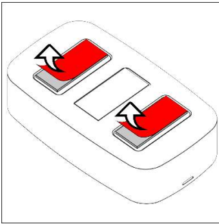
Şekil 7.1.1 – KB-1`in çift taraflı bantların takılması.
