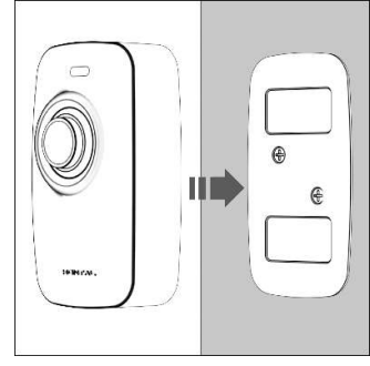
Şekil 7.2.3 – KB-1` in çift taraflı bant ile duvar montaj aparatına yapıştırılması.
