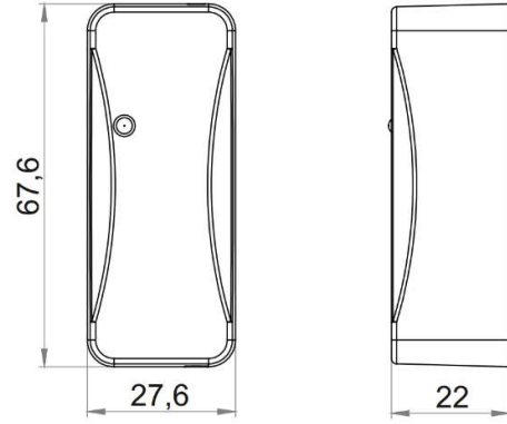
PESA Ölçüler (Birim; mm)
