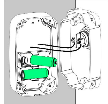
Şekil 7.3.3 – KB-1` in pil değişiminin yapılması.
