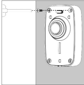
Şekil 7.3.2 – KB-1` in alt kapağının sökülmesi.
