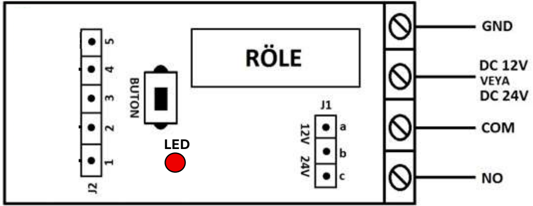
Şekil 8.1 PESA Bağlantı Şeması
