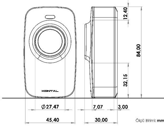
KB-1 Ölçüler (Birim; mm)
