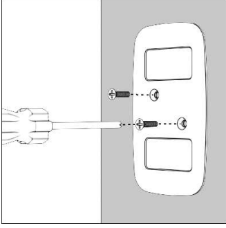
Şekil 7.2.1 – KB-1` in duvar montaj aparatının duvara vidalanması.
