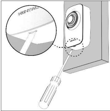
Şekil 7.3.1 – KB-1` in üst kapağının sökülmesi.
